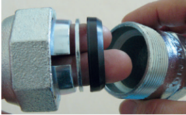
Bild 2: Konusmutter abschrauben, Klemmring und Vorlegering anheben und den Dichtring aus NBR herausnehmen und beiseite legen.
