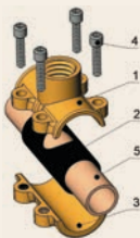
1 Oberteil Anbohrschelle mit Innengewinde-Abgang 2 Dichtmanschette 3 Unterteil Anbohrschelle 4 Inbusschraube 5 Rohr
